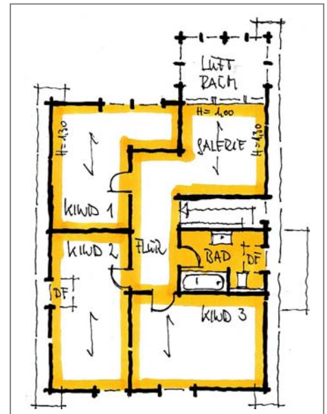
Obergeschoss 71,96 m 2
