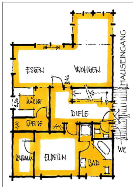
Erdgeschoss 94,93 m 2
